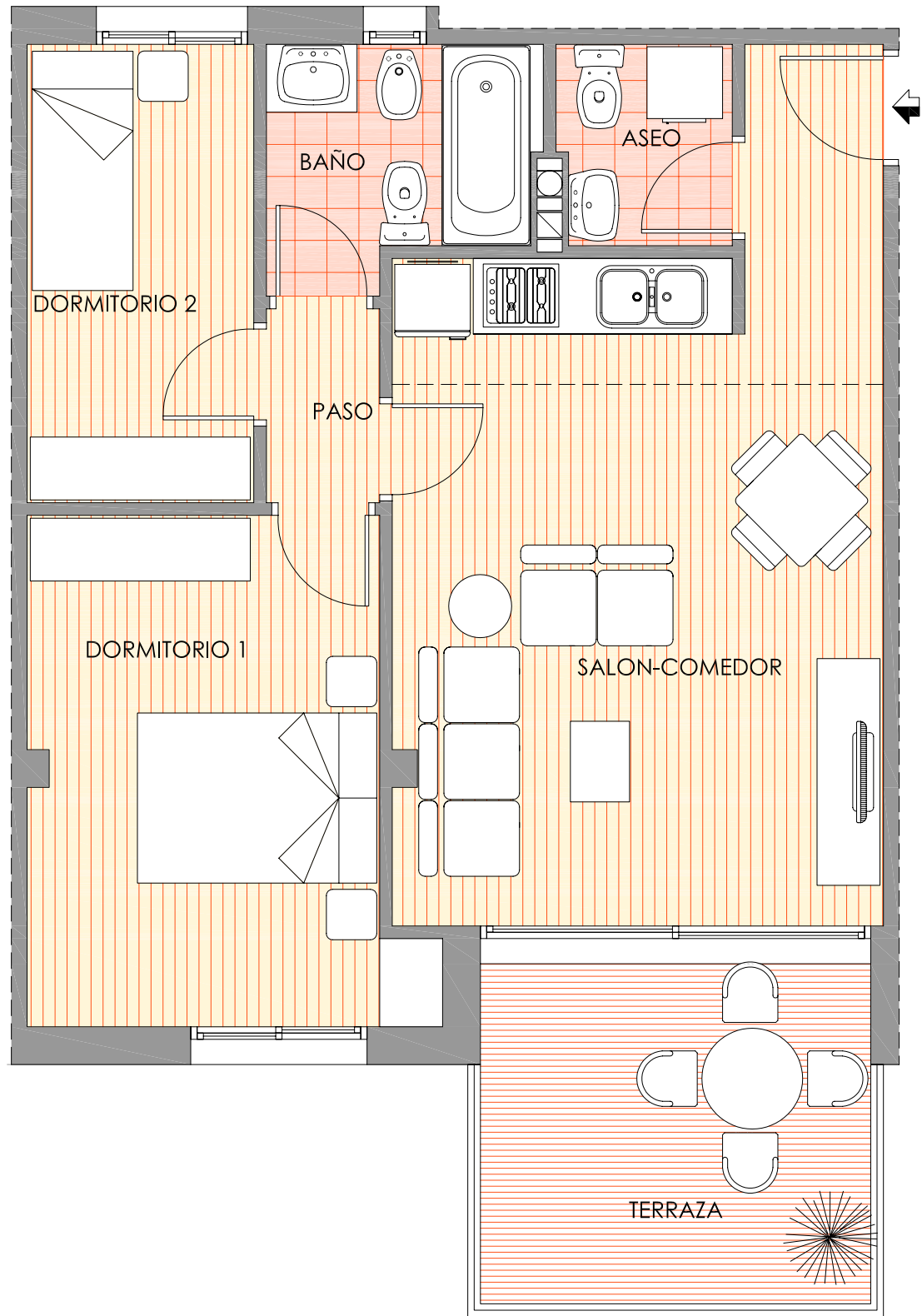
Vivienda Tipo "G-1" (Pl.1ª ) Escala 1/50
